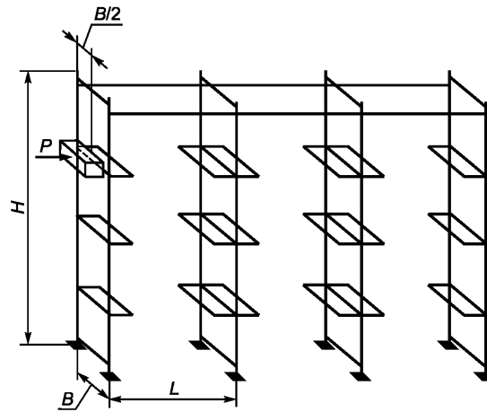
Глубинный стеллаж
