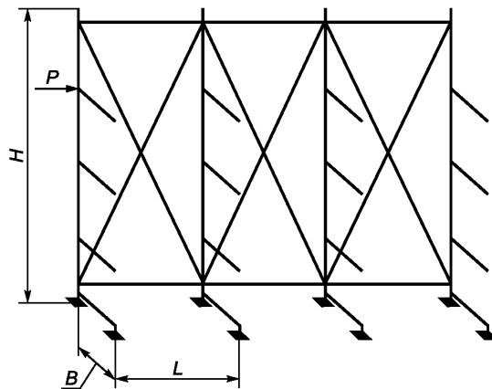
Консольный стеллаж
