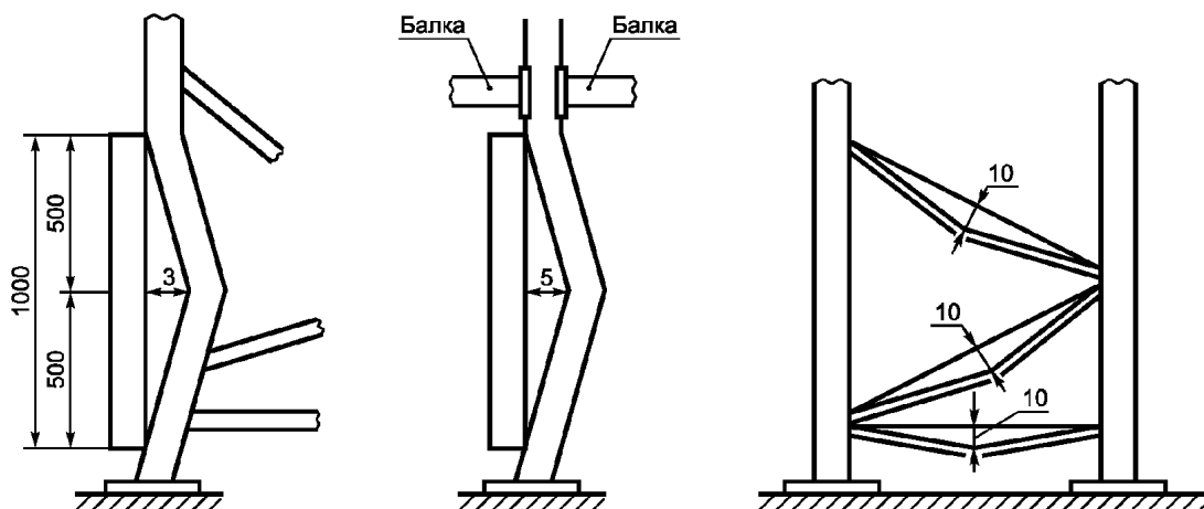
Рисунок Б.1 - Максимальные допустимые значения деформации
